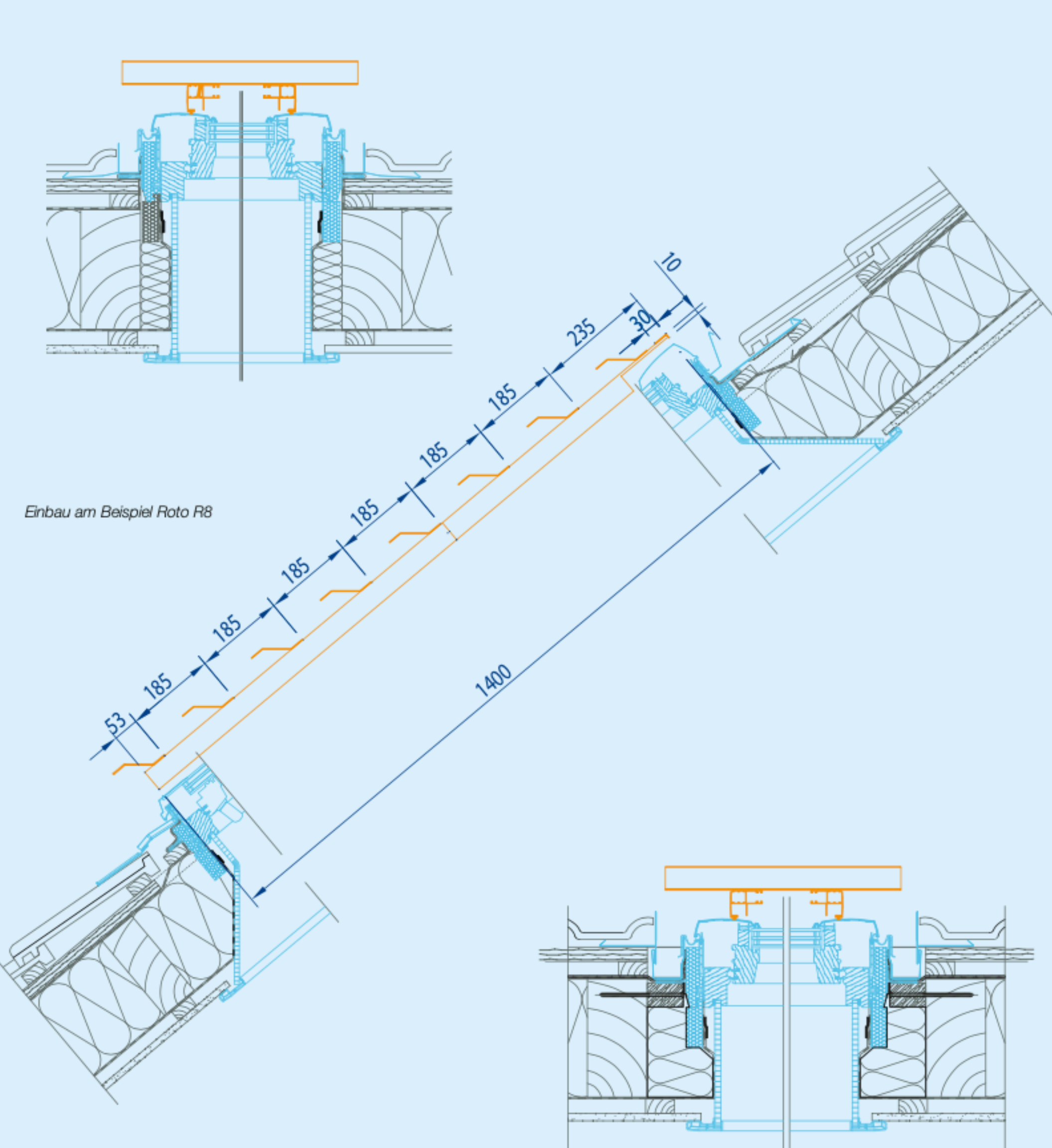
Beispiel vertiefter Einbau
