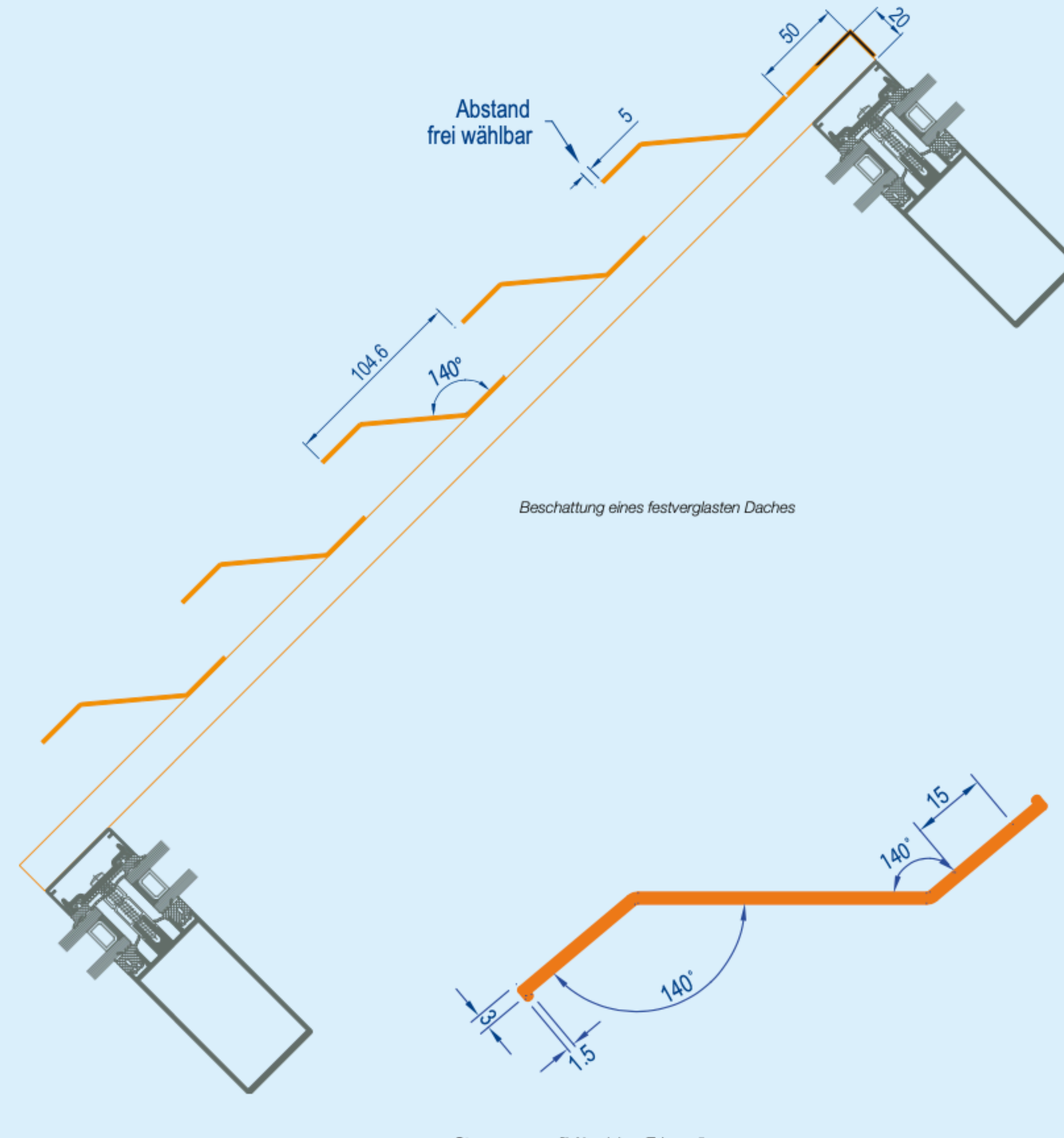
Strangpressprofil Aluminium Z-Lamelle
