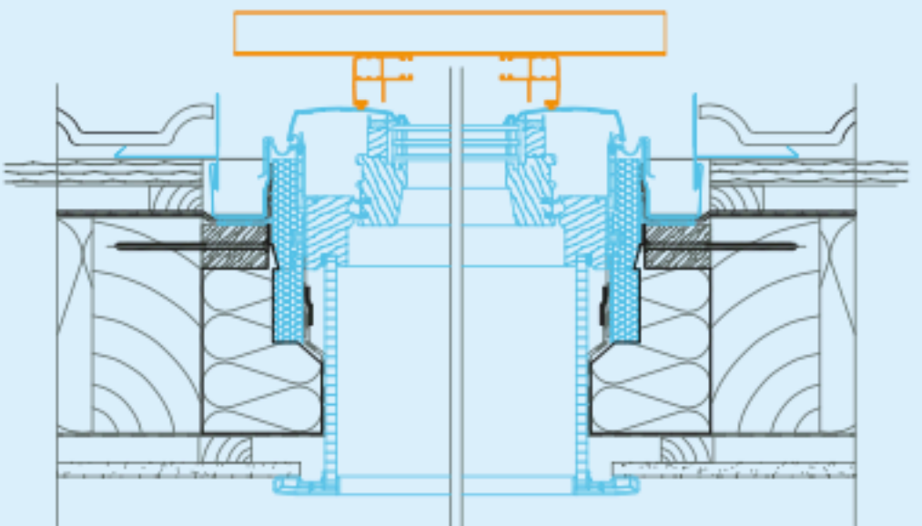
Beispiel vertiefter Einbau
